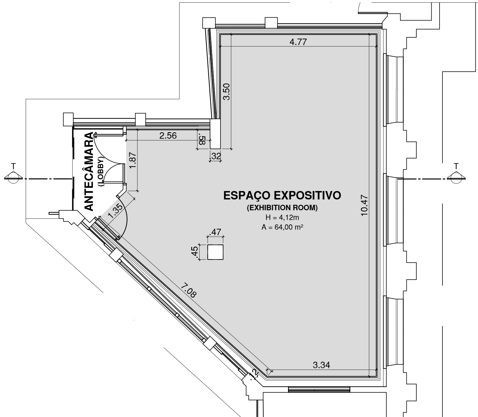
PLANTA DO 3º ANDAR (3rd FLOOR PLAN)
