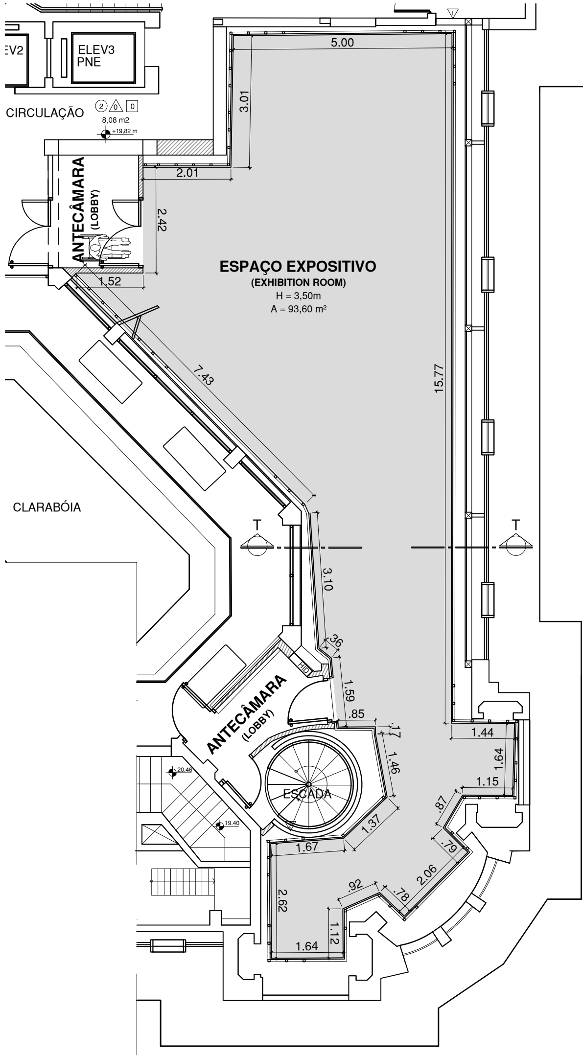
PLANTA DO 4º ANDAR (4th FLOOR PLAN)
